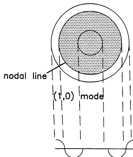
(1,0) mode FIG. 2b
