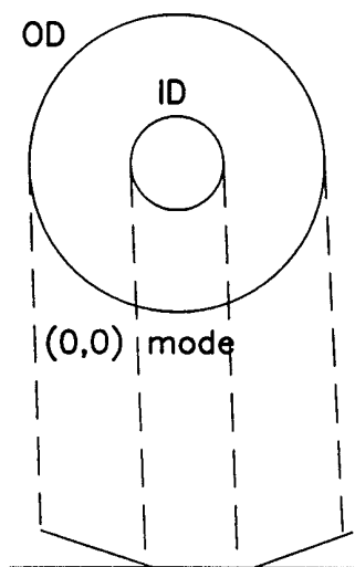
(0,0) mode FIG. 2a
