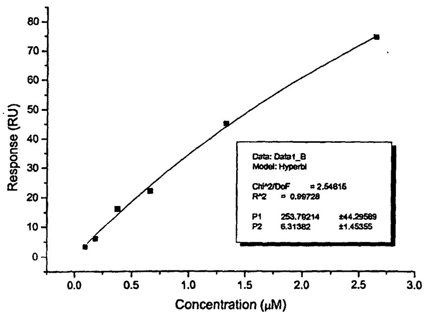
Figure 82: Ser 15/Glu 15
