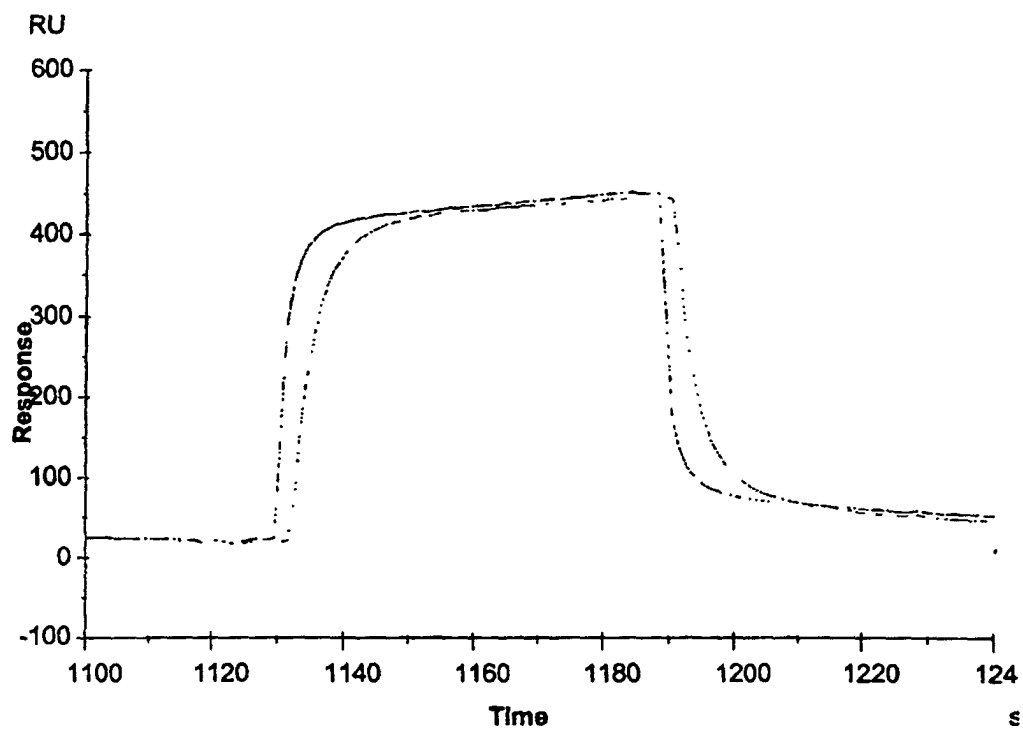
Figure 81: Met 52/Gly 55
