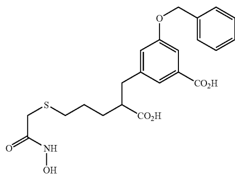
3-Benzyloxy-5-(2-carboxy-5-hydroxycarbonylmethylsulfanyl)pentyl)-benzoic acid
