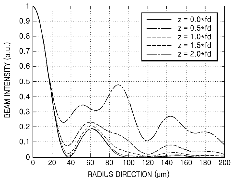
FIG. 20C
