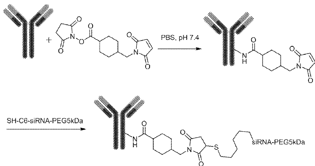
Conjugation Scheme-2
