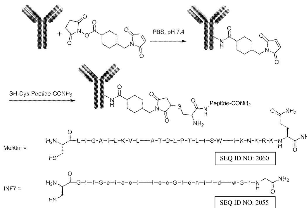
Conjugation Scheme-4
