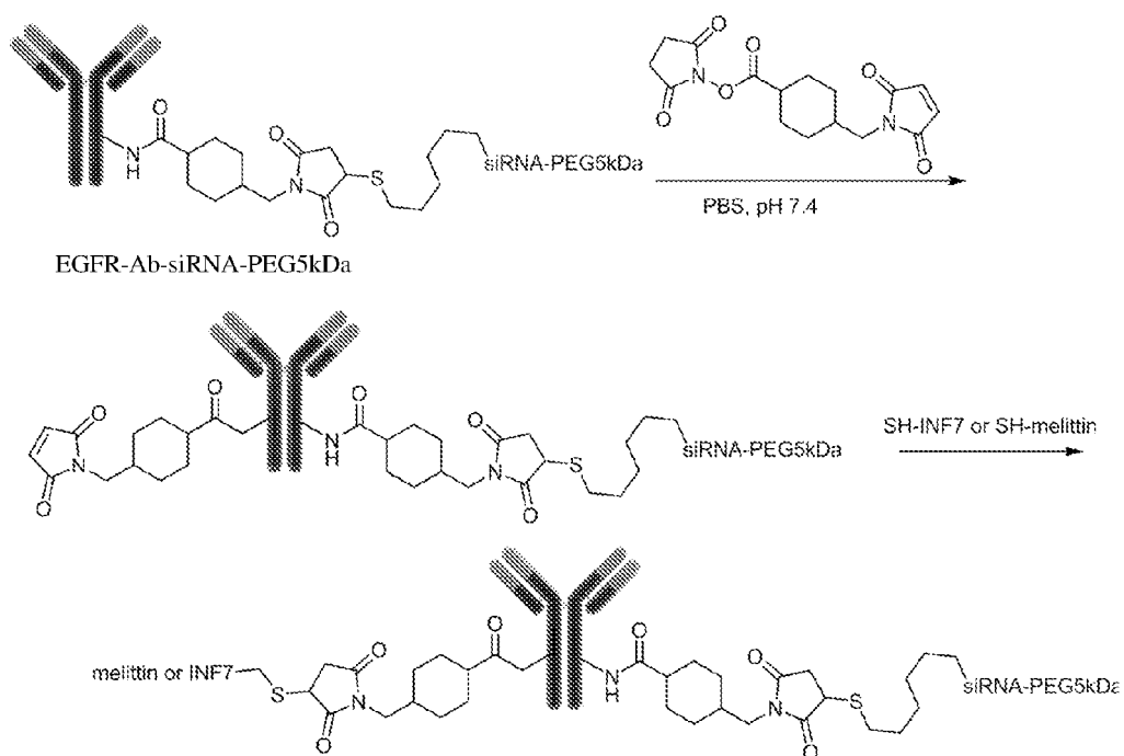
Conjugation Scheme-5
