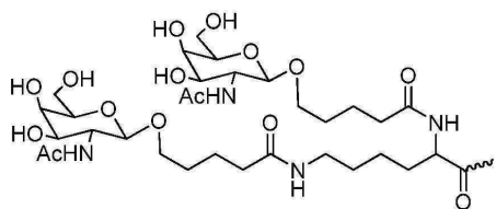
화학식 XVI,
