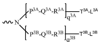
화학식 XXXII
