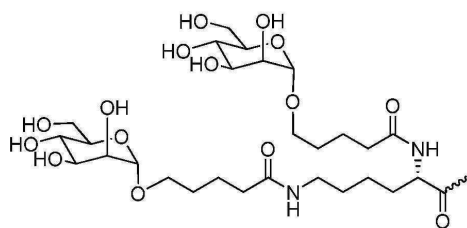
화학식 XXI,
