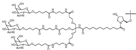
(화학식 XXIV),
