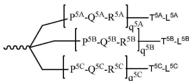
화학식 XXXIV
