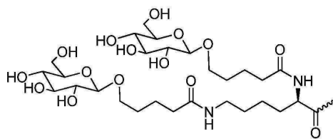
화학식 XVIII,
