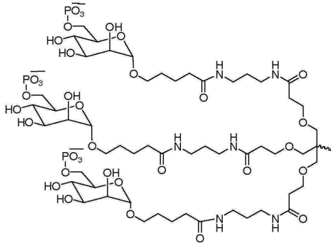
화학식 XI,
