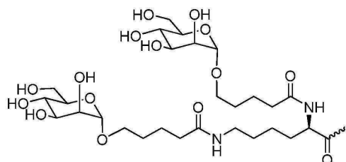
화학식 XXII
