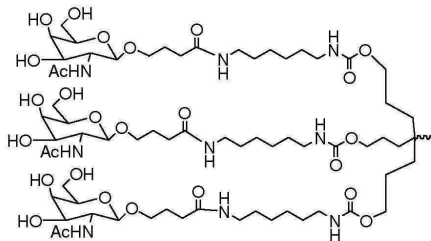
화학식 XIII,
