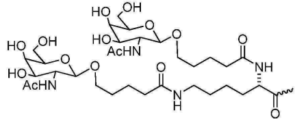
화학식 XIV,
