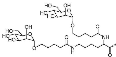
화학식 XX,
