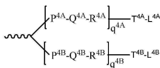
화학식 XXXIII
