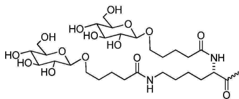
화학식 XVII,
