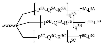
화학식 XXXV
