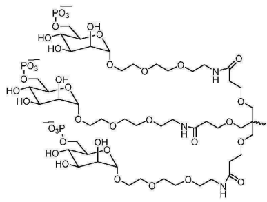
화학식 XI,
