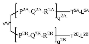
화학식 XXXI
