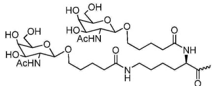
화학식 XV,
