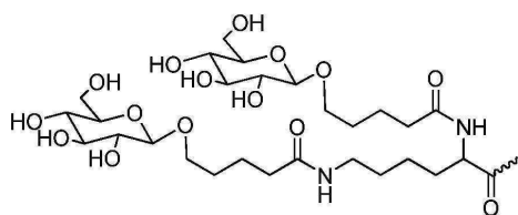
화학식 XIX,
