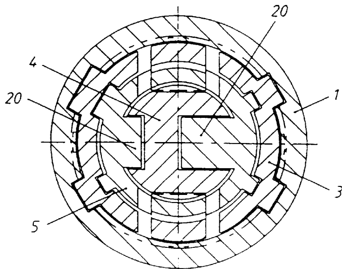
Fig. 6 section B-B
