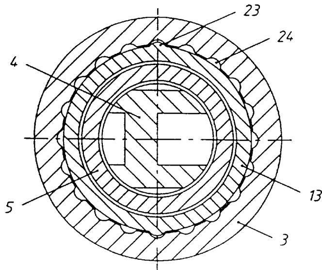
Fig. 5 section A-A
