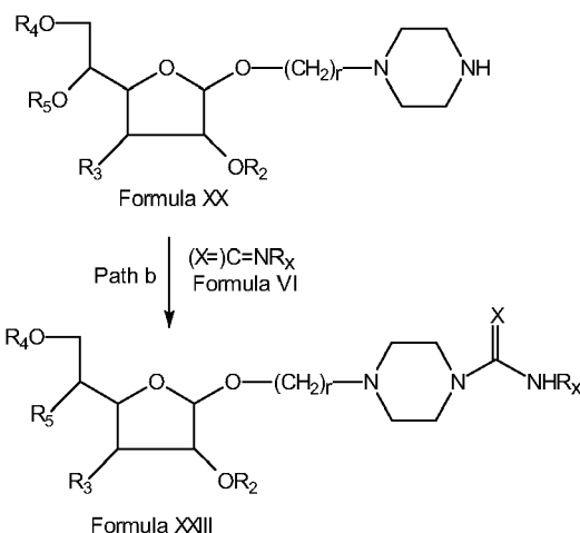
SCHEME VI
