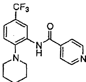
SRPIN-1(C 18 H 18 F 3 N 3 O) MW349.35
