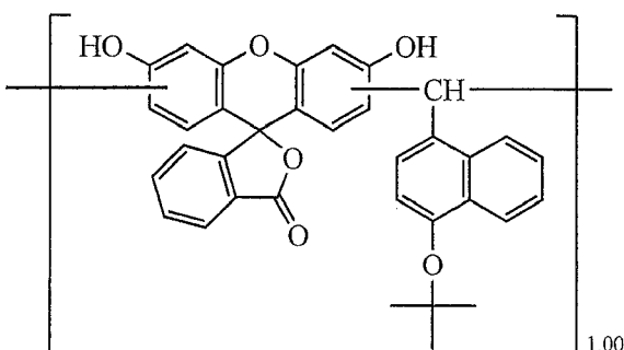
Novolak Resin 17
