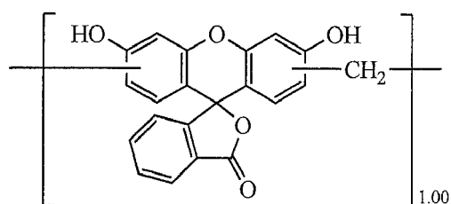
Novolak Resin 2
