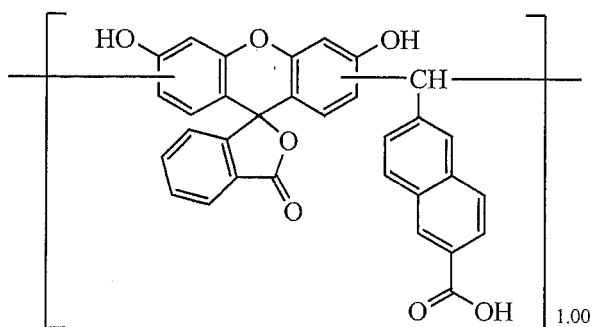
Novolak Resin 14
