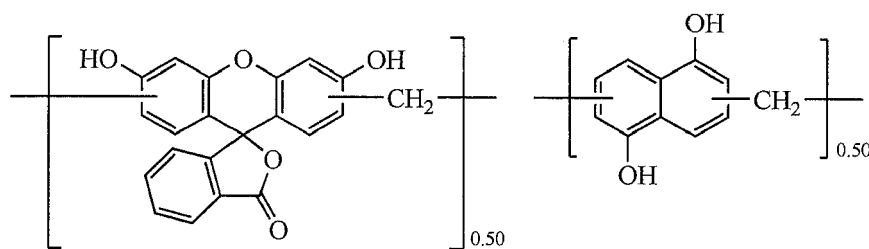
Novolak Resin 4
