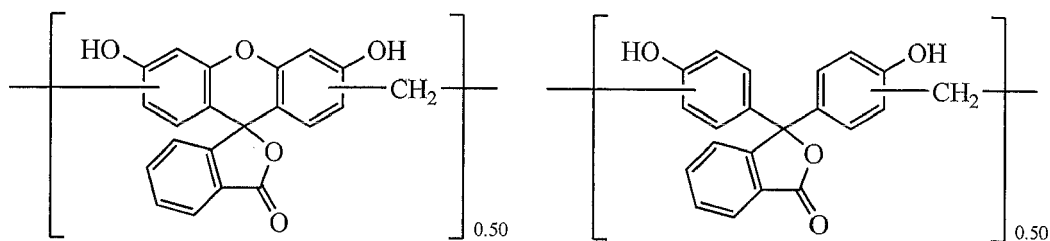
Novolak Resin 11
