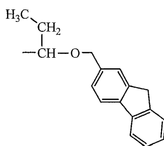
(A-2)-68
