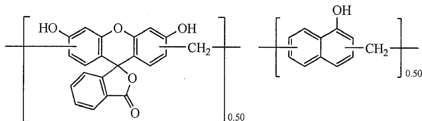
Novolak Resin 3
