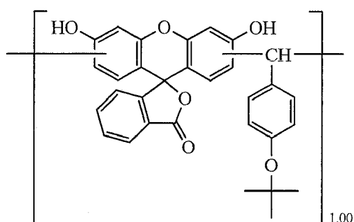
Novolak Resin 18
