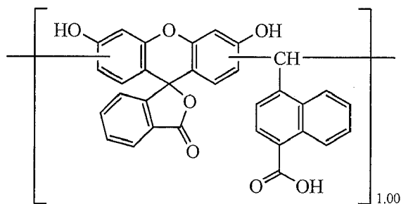
Novolak Resin 16
