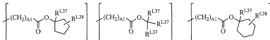
(A-1)-1
