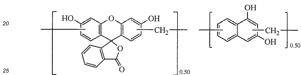
Novolak Resin 5
