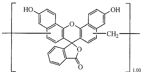
Novolak Resin 13
