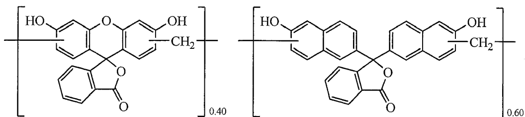
Novolak Resin 9
