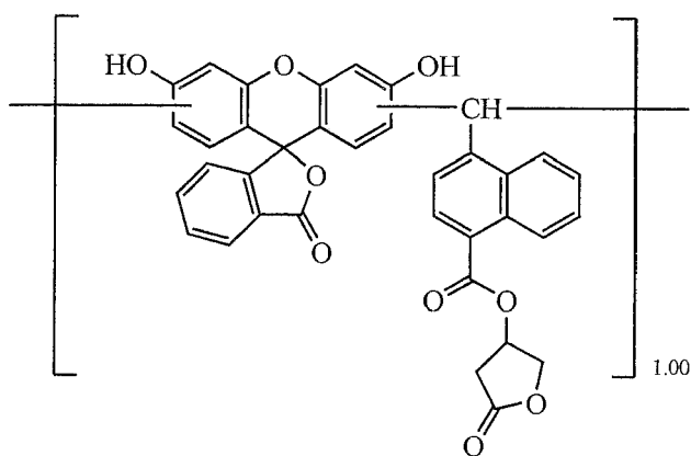
Novolak Resin 15
