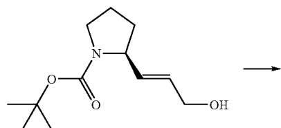
Scheme VI
