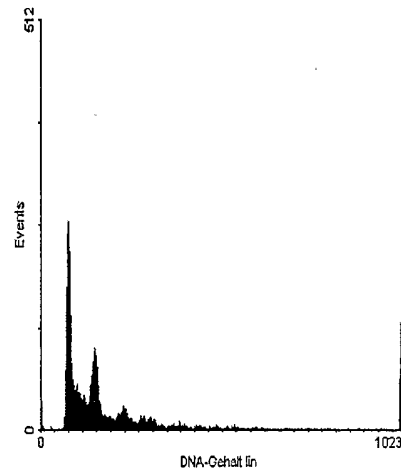
DNA-Gehalt
