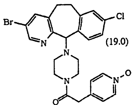
(-)-对映体 ;
