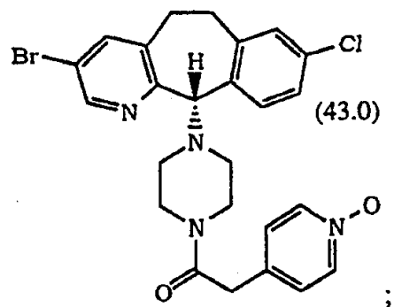
(+) - 对映体
