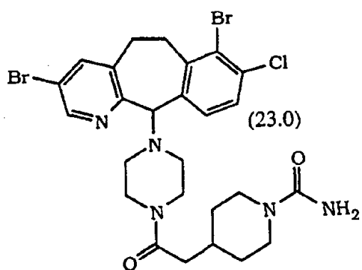
(-)-对映体 ;
