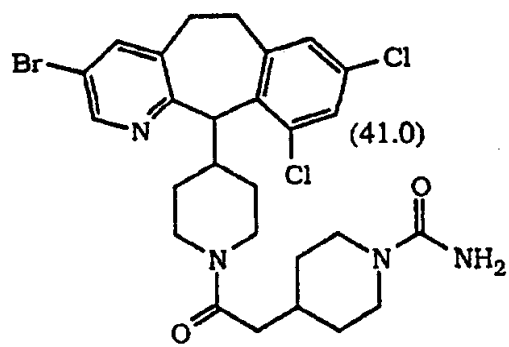
(+) - 对映体
