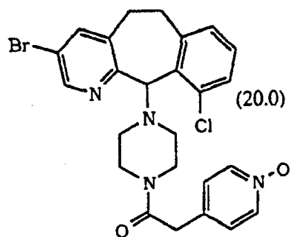
(+) -对映体 ;
