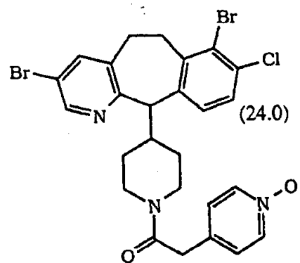
(+) -对映体 ;
