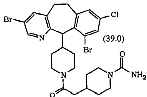
(+) -对映体 ;
