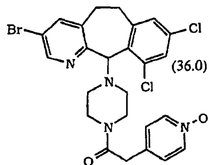
(+) -对映体 ;
