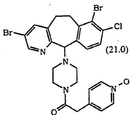
(+) -对映体 ;
