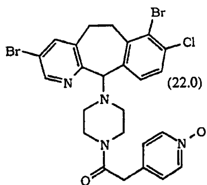
(-)-对映体 ;
