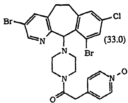
(-)-对映体 ;
