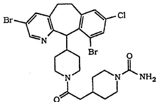
(+)-对映体
