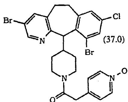
(+) -对映体 ;
