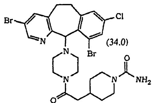
(+) -对映体 ;
