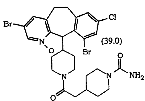
(+)-对映体
