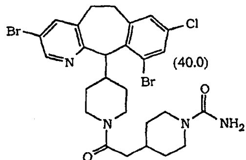
(-)-对映体 ;
