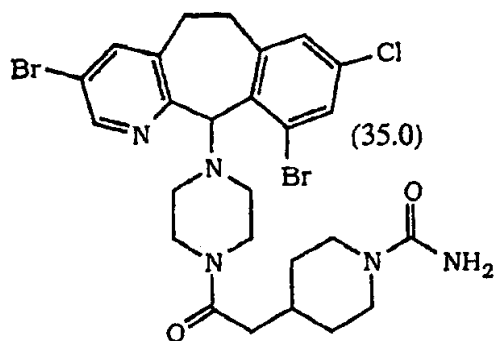
(-)-对映体 ;
