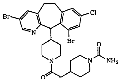
(+)-对映体
