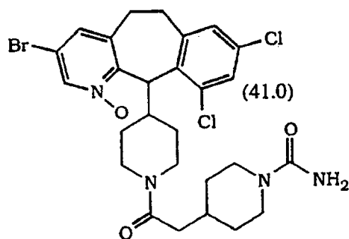
(+)-对映体
