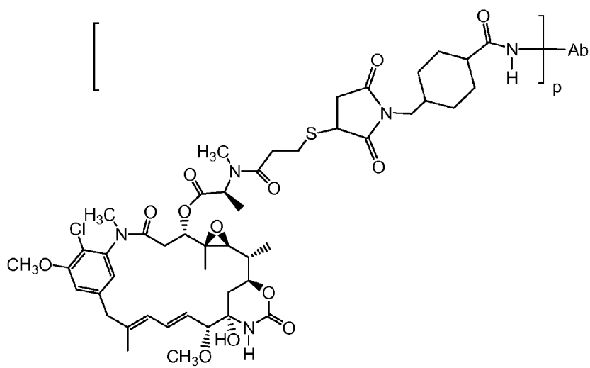
Ab-SPDB-DM4
