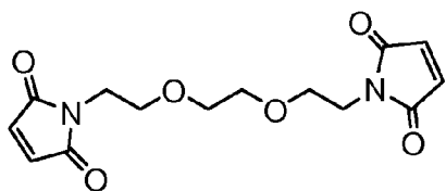
BM(PEO) 2
