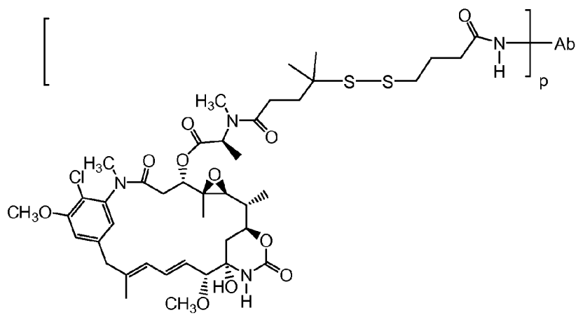
Ab-SPDB-DM4
