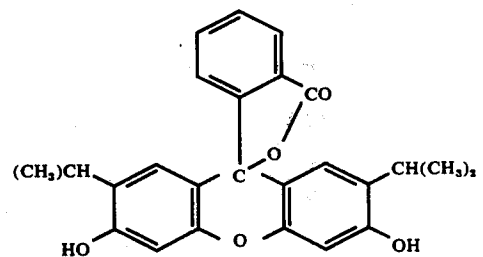
Compound VIII-4
