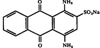
Compound VII-4
