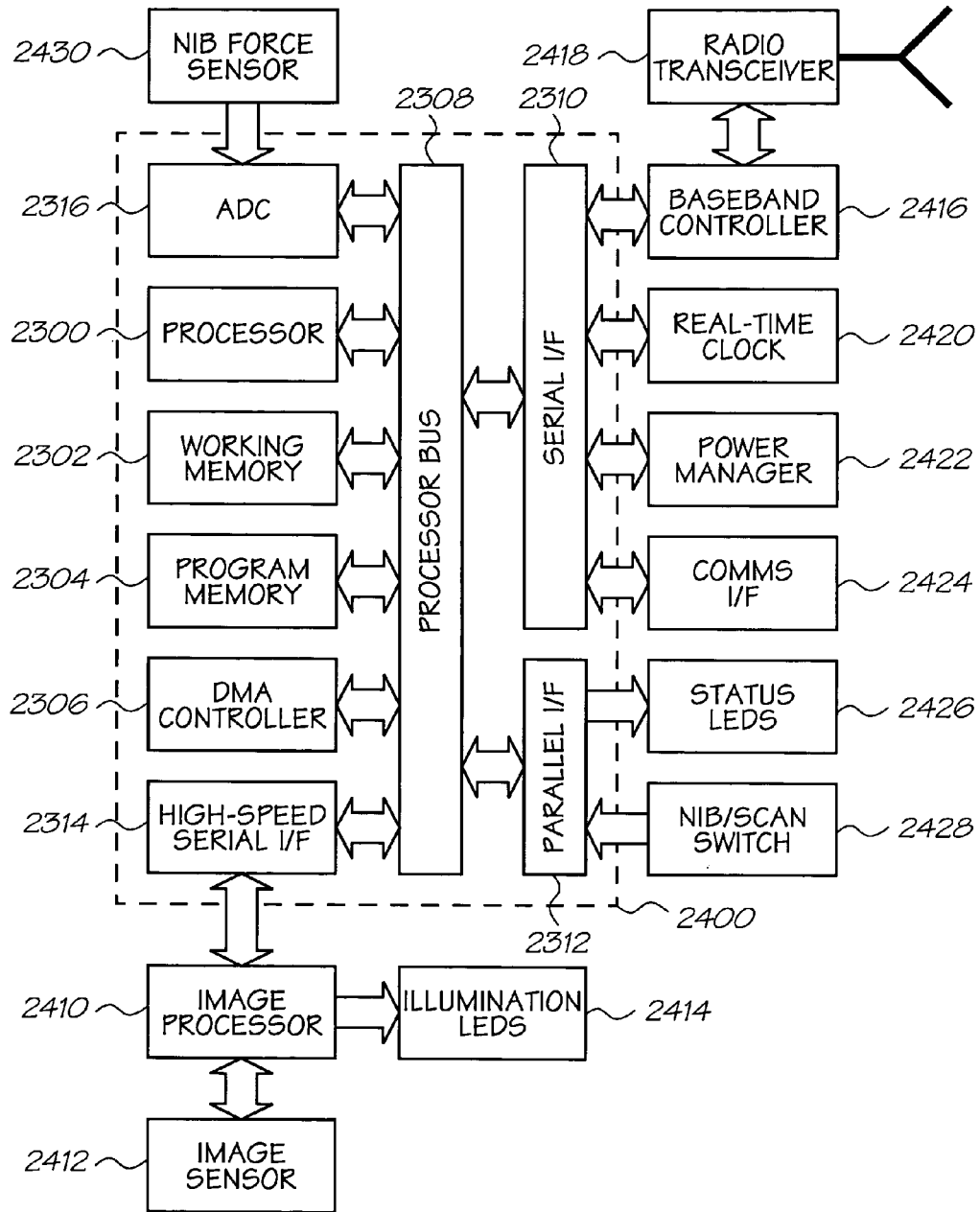
FIG. 69
