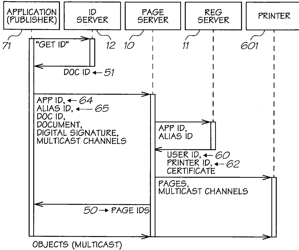
FIG. 40
