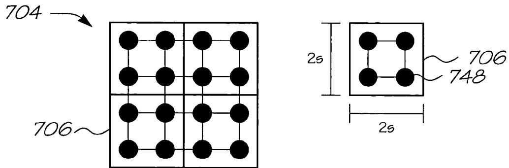
FIG. 45
