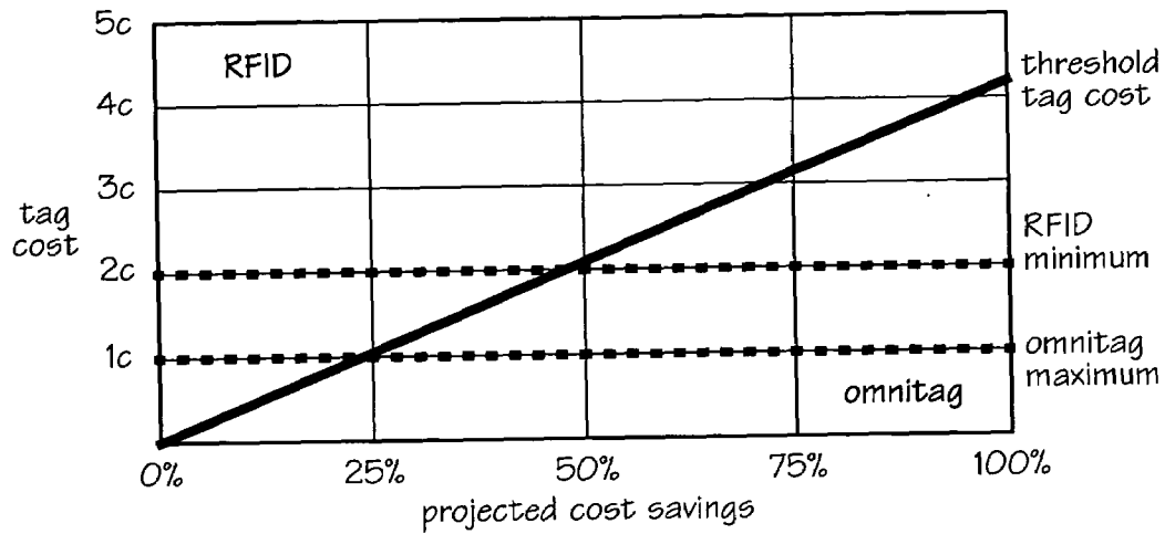
FIG. 97
