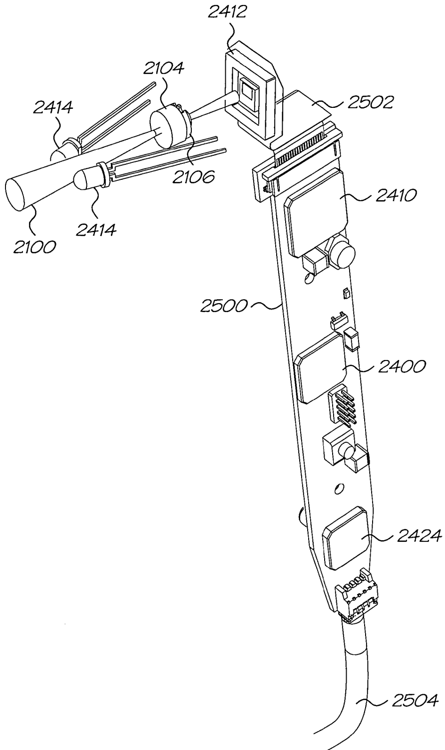
FIG. 62
