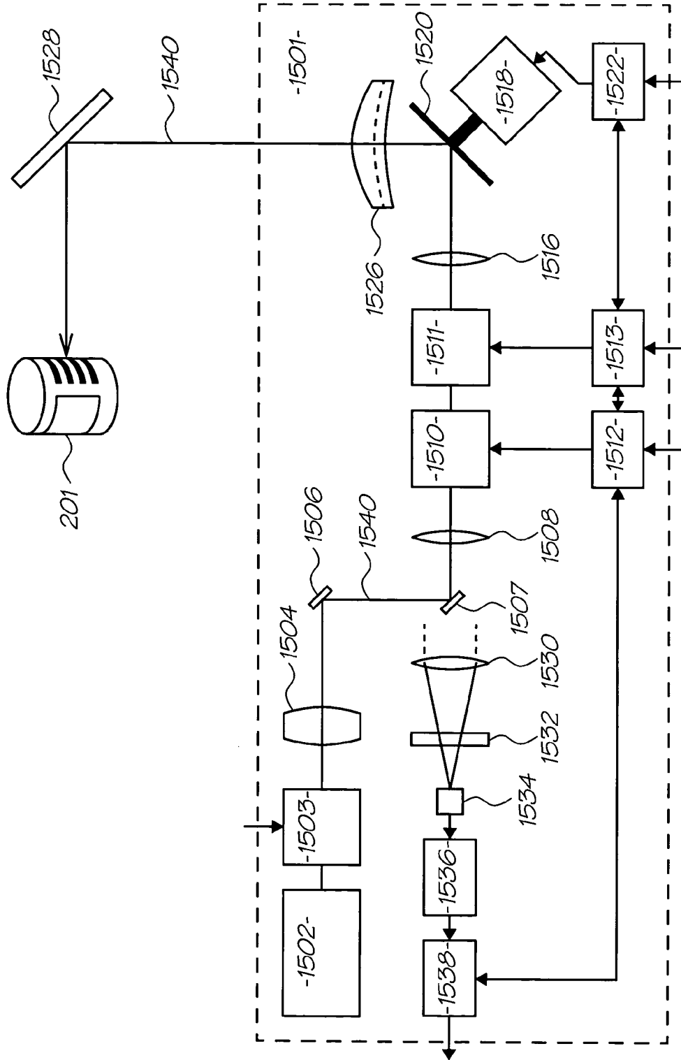
FIG. 76
