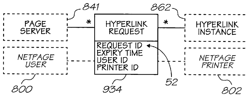
FIG. 41
