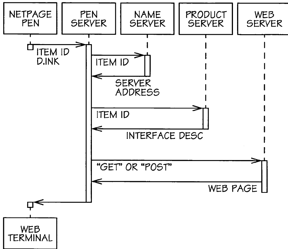
FIG. 99
