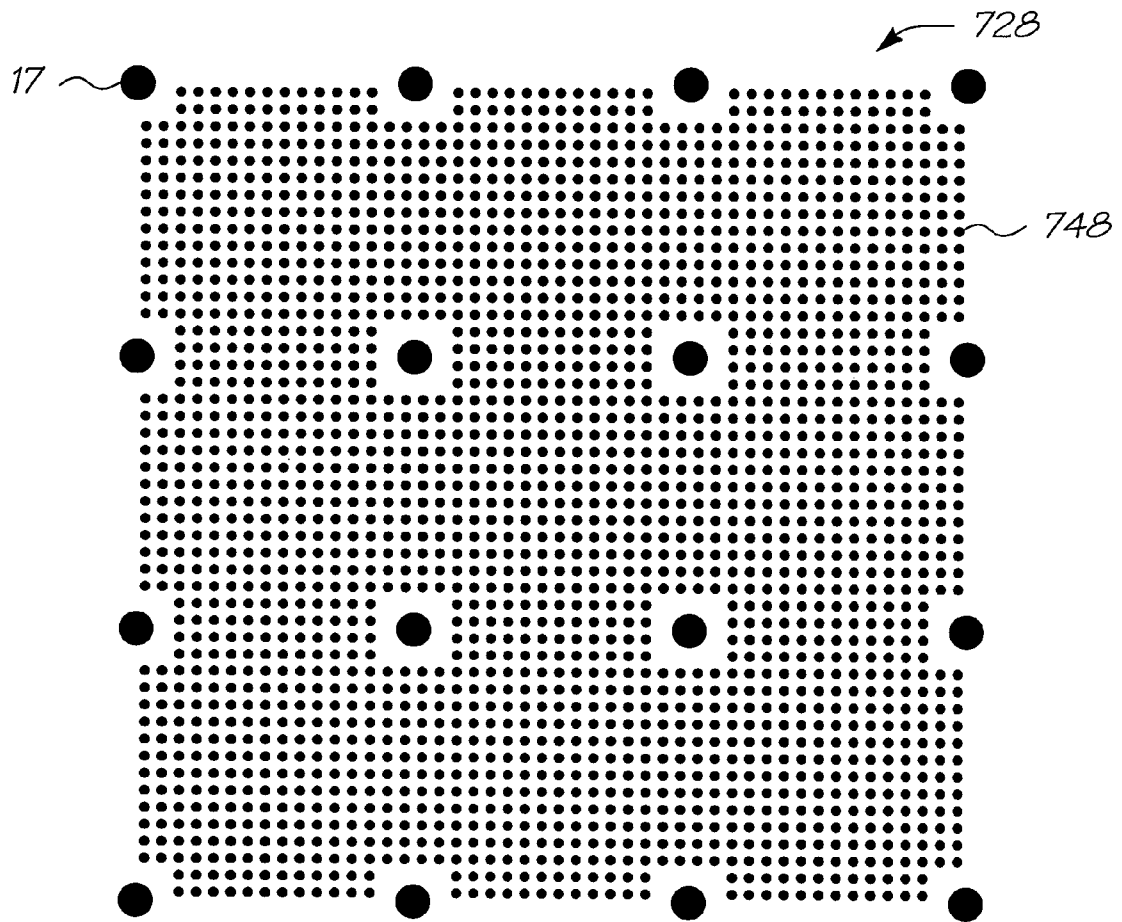
FIG. 5c
