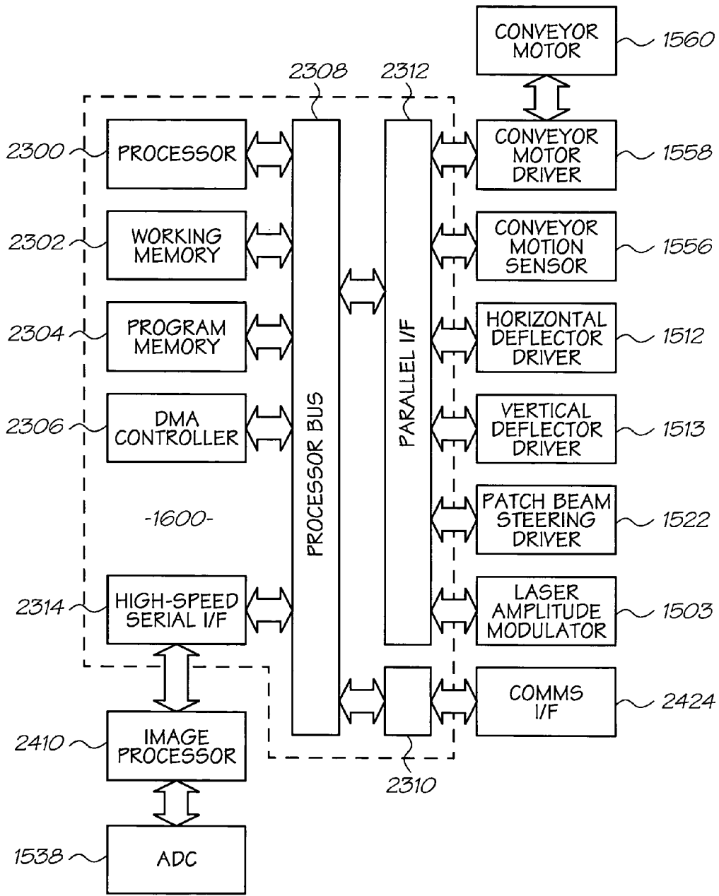
FIG. 85
