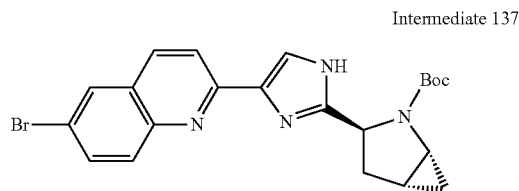
tert-Butyl (1R,3S,5R)-3-(4-(6-bromo-2-quinolinyl)-1H-imidazol-2-yl)-2-azabicyclo[3.1.0]hexane-2-carboxylate
