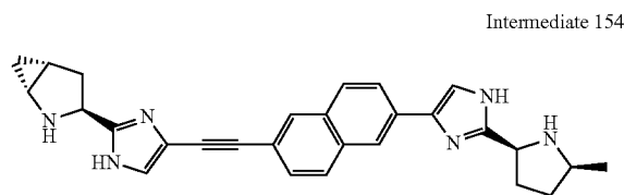
(1R,3S,5R)-3-(4-(((6-(2-((2S,5S)-5-Methylpyrrolidin-2-yl)-1H-imidazol-4-yl)naphthalen-2-yl)ethynyl)-1H-imidazol-2-yl)-2-azabicyclo[3.1.0]hexane
