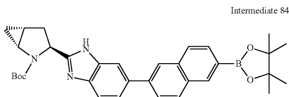
(1R,3S,5R)-tert-Butyl 3-(6-(6-(4,4,5,5-tetramethyl-1,3,2-dioxaborolan-2-yl)naphthalen-2-yl)-1H-benzo[d]imidazol-2-yl)-2-azabicyclo[3.1.0]hexane-2-carboxylate
