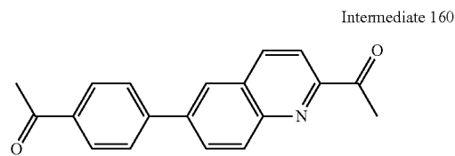
1-(6-(4-Acetylphenyl)quinolin-2-yl)ethanone
