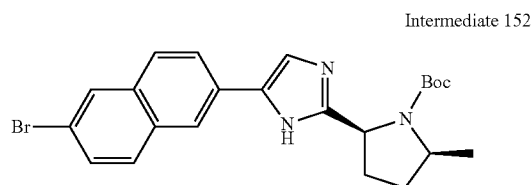
(2S,5S)-tert-Butyl 2-(5-(6-bromonaphthalen-2-yl)-1H-imidazol-2-yl)-5-methylpyrrolidine-1-carboxylate
