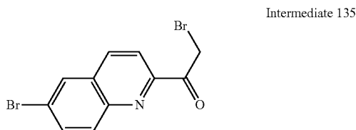
2-Bromo-1-(6-bromoquinolin-2-yl)ethanone
