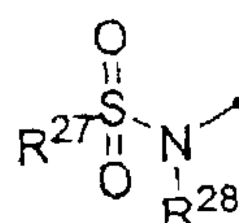
Sulfonamido group
