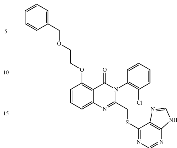
5-(2-Benzyloxyethoxy)-3-(2-chlorophenyl)-2-(9H-purin-6-ylsulfanylmethyl)-3H-quinazolin-4-one (D-078)
