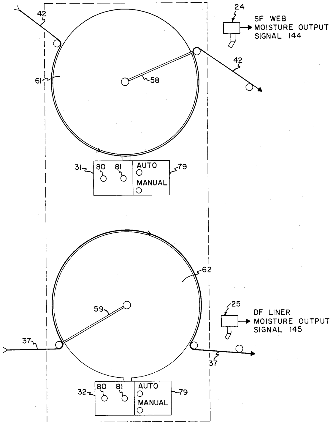
SF WEB & DF PREHEATERS & WRAP ARMS
