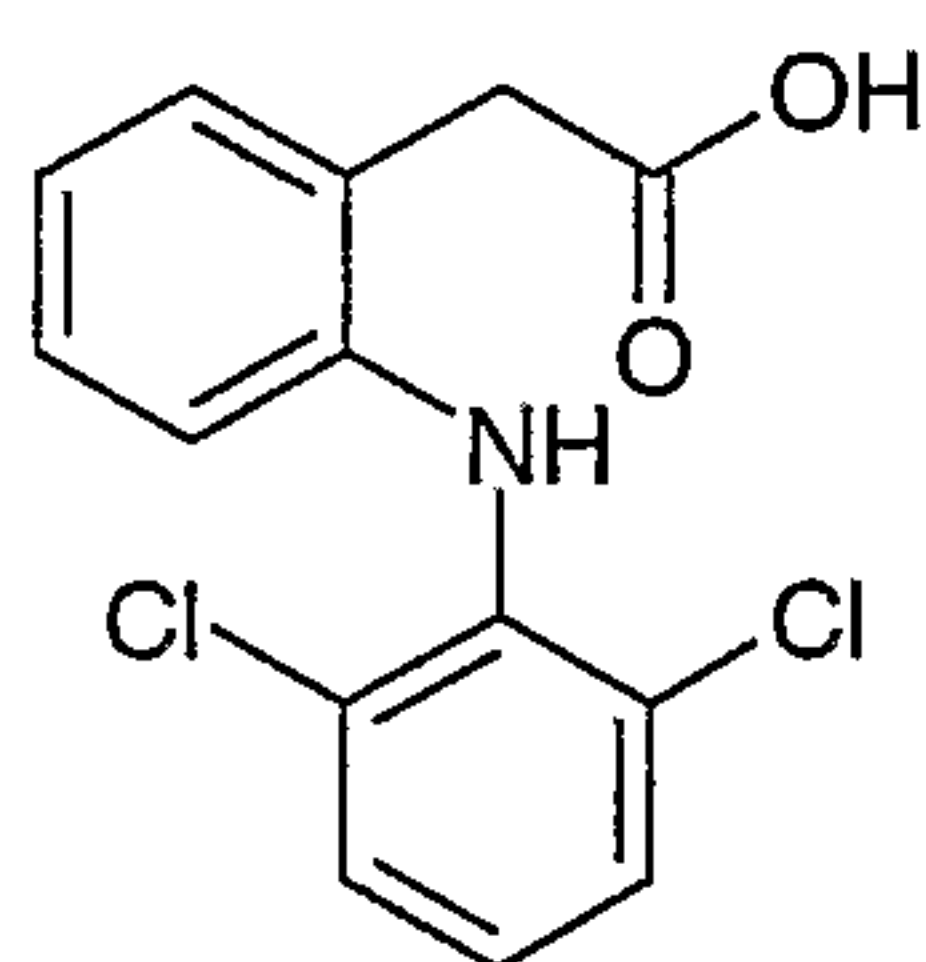
Diclofenac (Ia)
