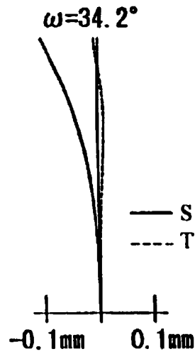
Astigmatism Fig. 10(B)
