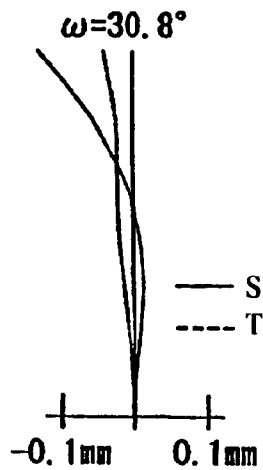
Astigmatism Fig. 7(B)
