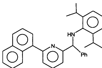
Precursor Z
