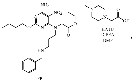
Scheme 107:
