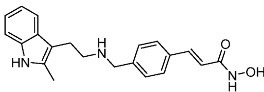
Panobinostat
