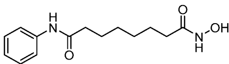
SAHA
