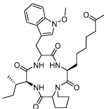
Apicidin
