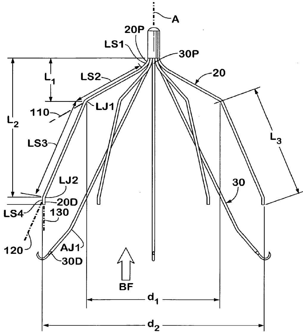
FIG.4A
