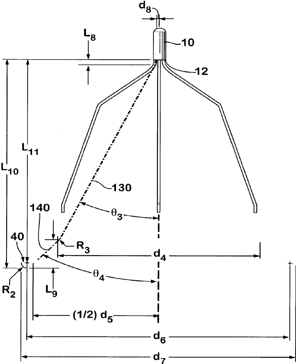
FIG.5B
