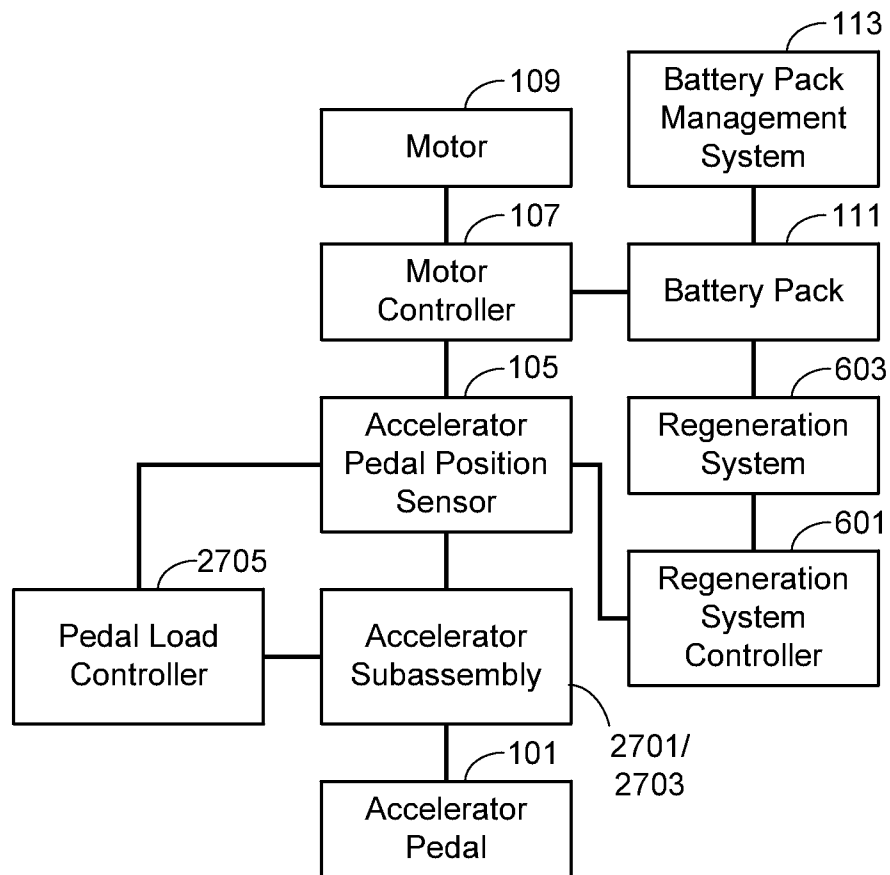
FIG. 29
