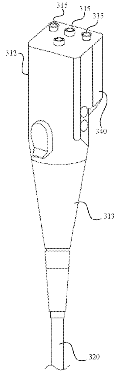
FIG. 7C
