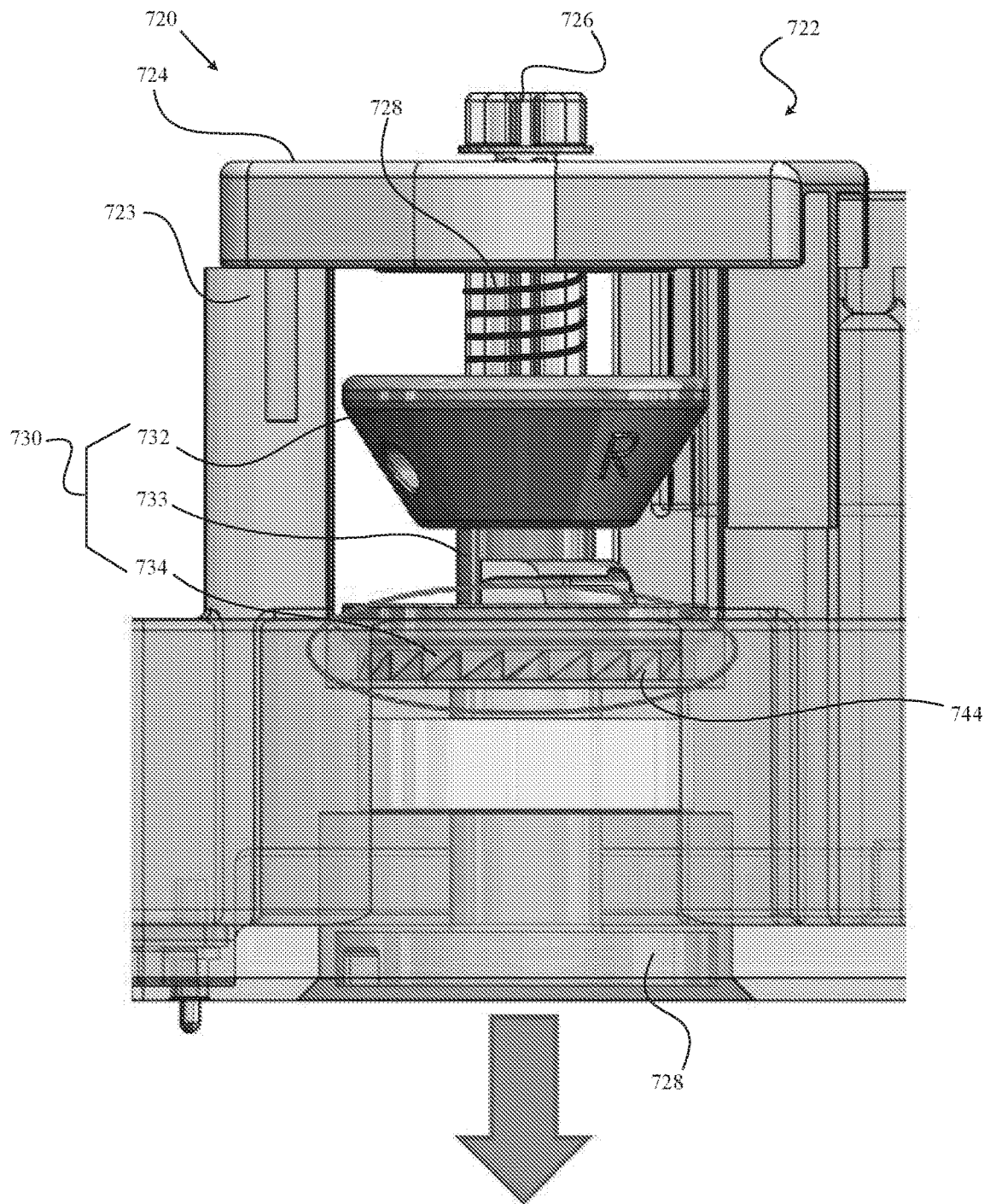
FIG. 18D
