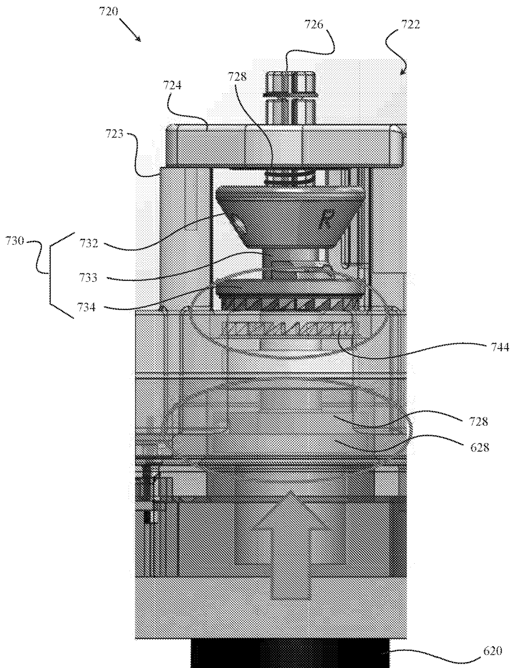
FIG. 18C
