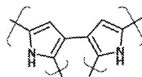
\beta, \beta'
