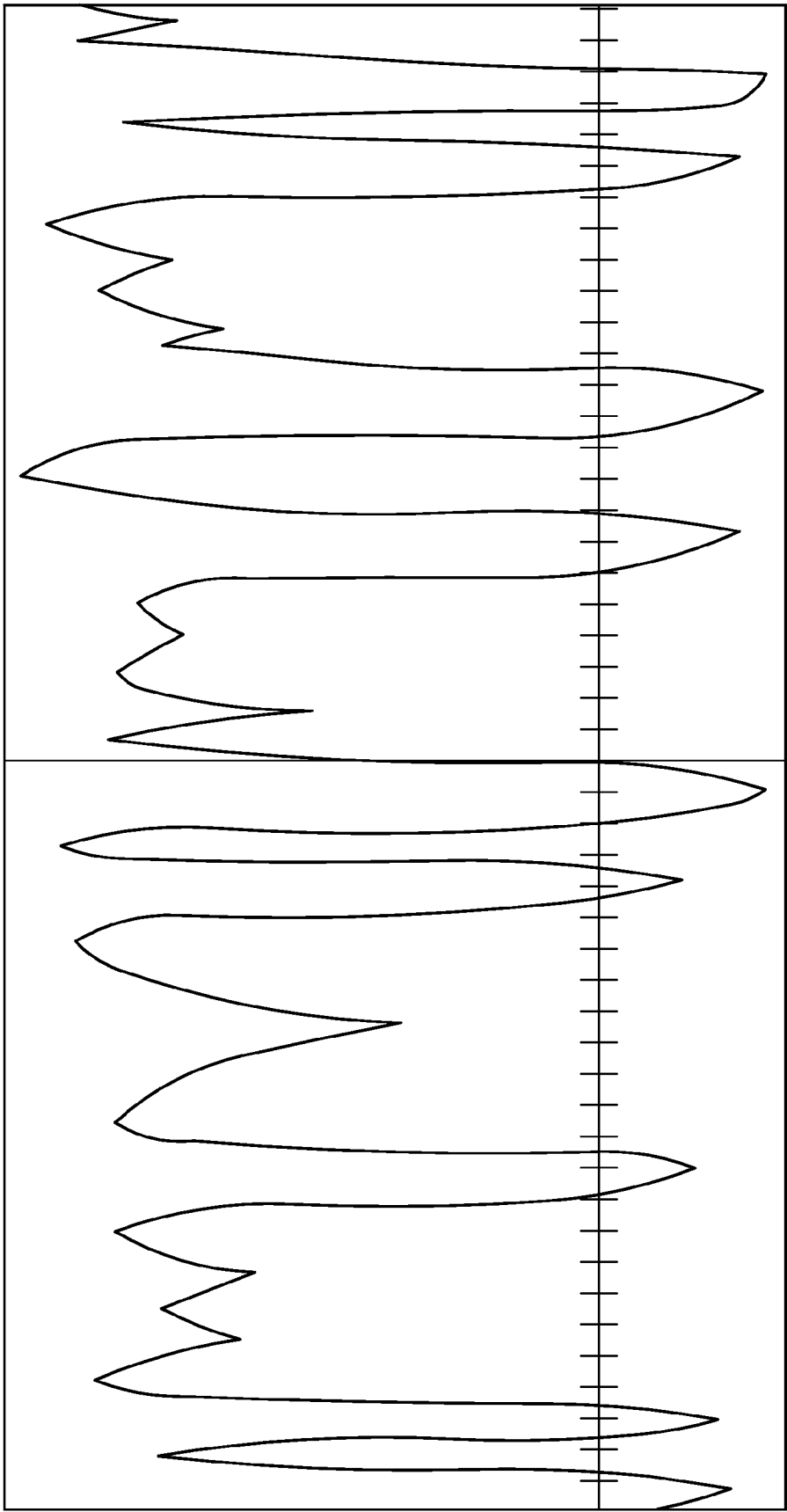
ACTUAL CVR VIDEO SIGNAL
