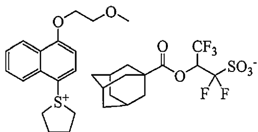
PAG-2
