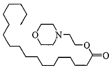
Q-3
