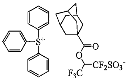
PAG-1
