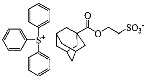
Q-1
