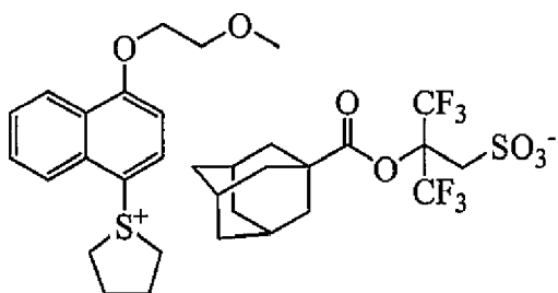
PAG-3
