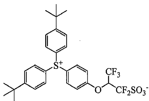
PAG-4
