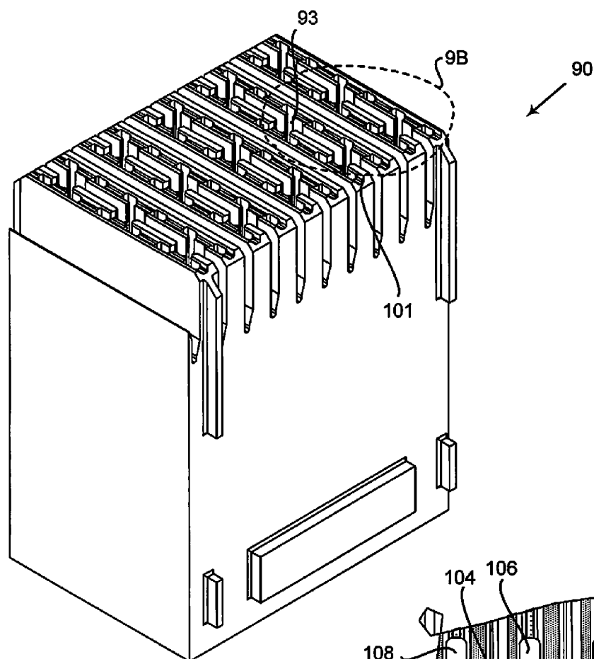
FIGURE 9A
