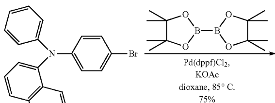
N-(4-bromophenyl)-N-phenylnaphthalen-1-amine
