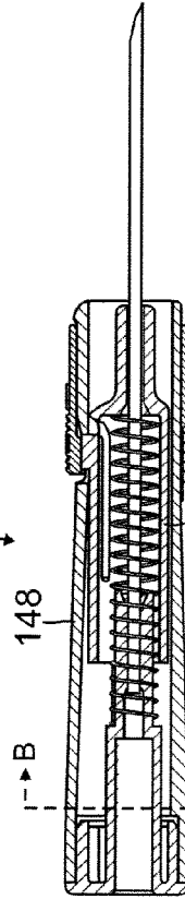
FIG. 16 SECTION A-A
