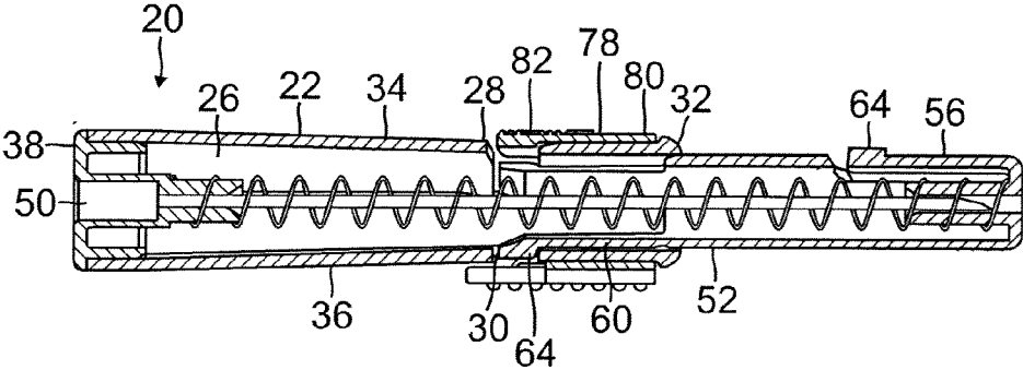
FIG. 6 SECTION D-D
