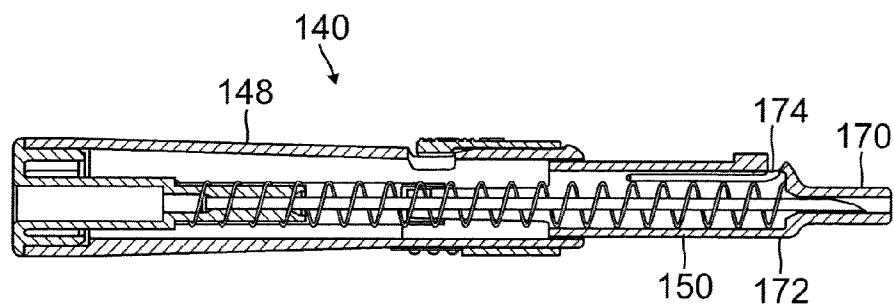
FIG. 19 SECTION D-D
