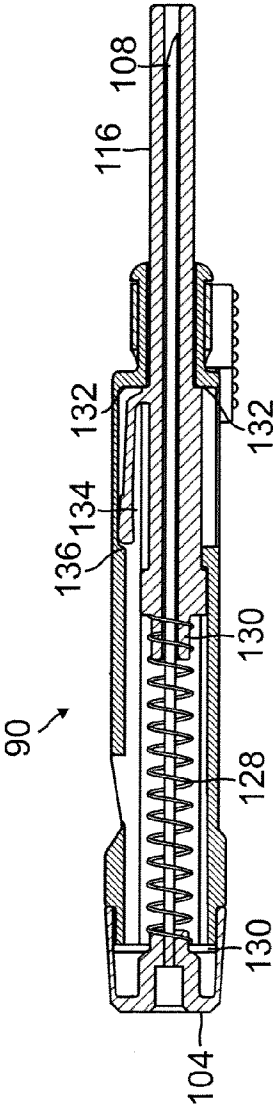
FIG. 12 SECTION D-D
