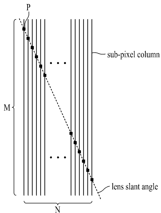
FIG. 19A
