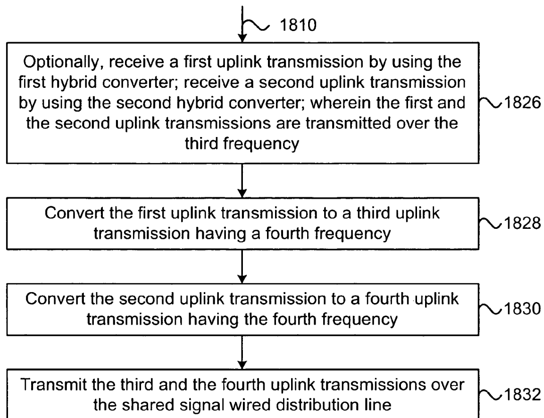
FIG. 18D
