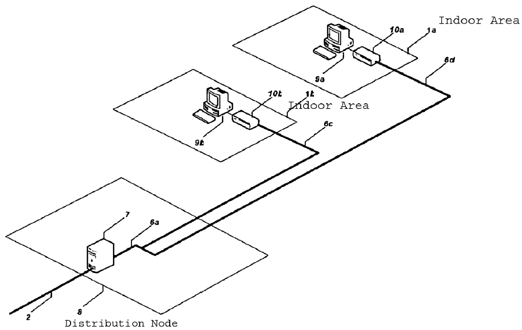
FIG. 1F
