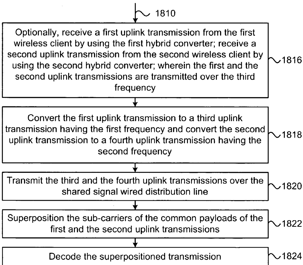
FIG. 18C
