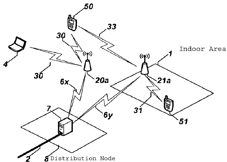
FIG. 1G
