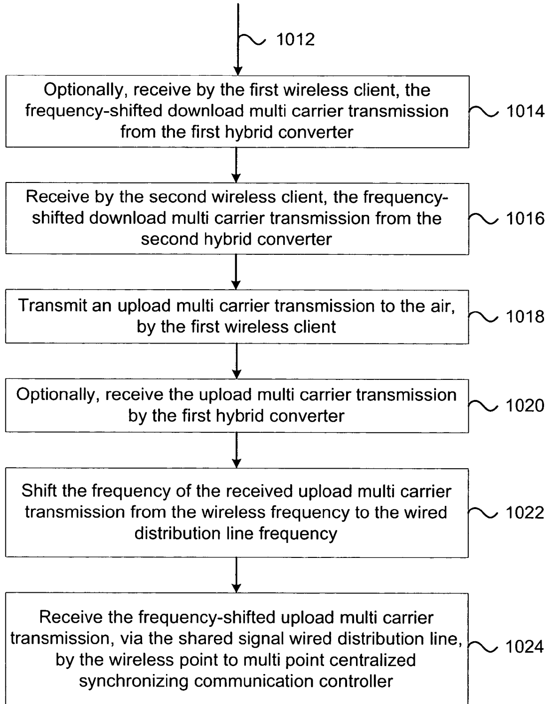
FIG. 10B
