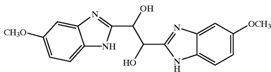
1,2-(5-methoxy-2-benzimidazole)-1,2-ethanediol
