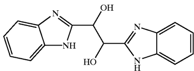
1,2-bis(2-benzimidazole)-1,2-ethanediol
