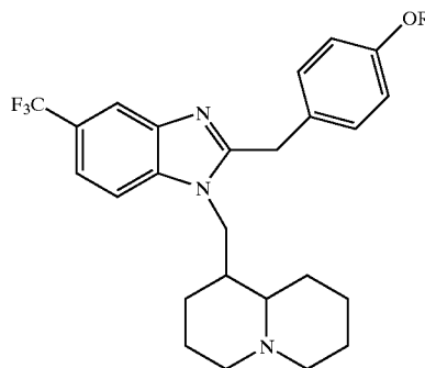
2-Benzyl-benzimidazole
