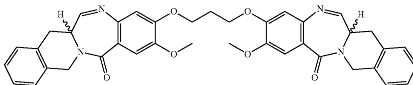
1 CLT-D201
