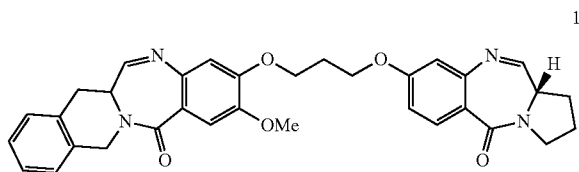
CLT-D501
