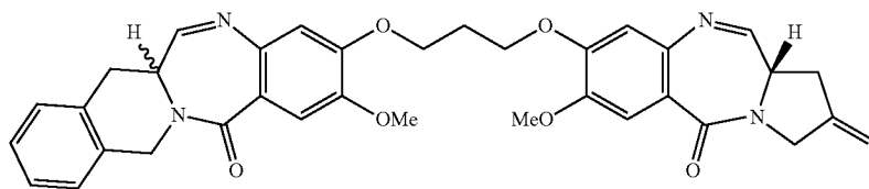
CLT-D601
