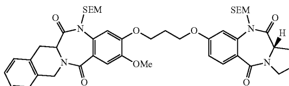
Bis-SEM-CLT-D501
