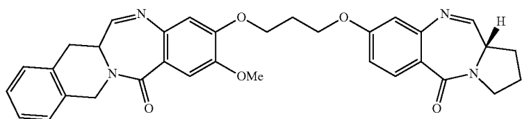
CLT-D501
