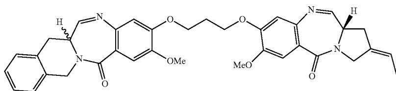
CLT-D601
