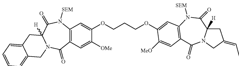
Bis-SEM CLT-D601
