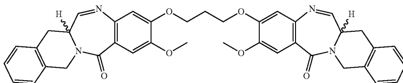
CLT-D201
