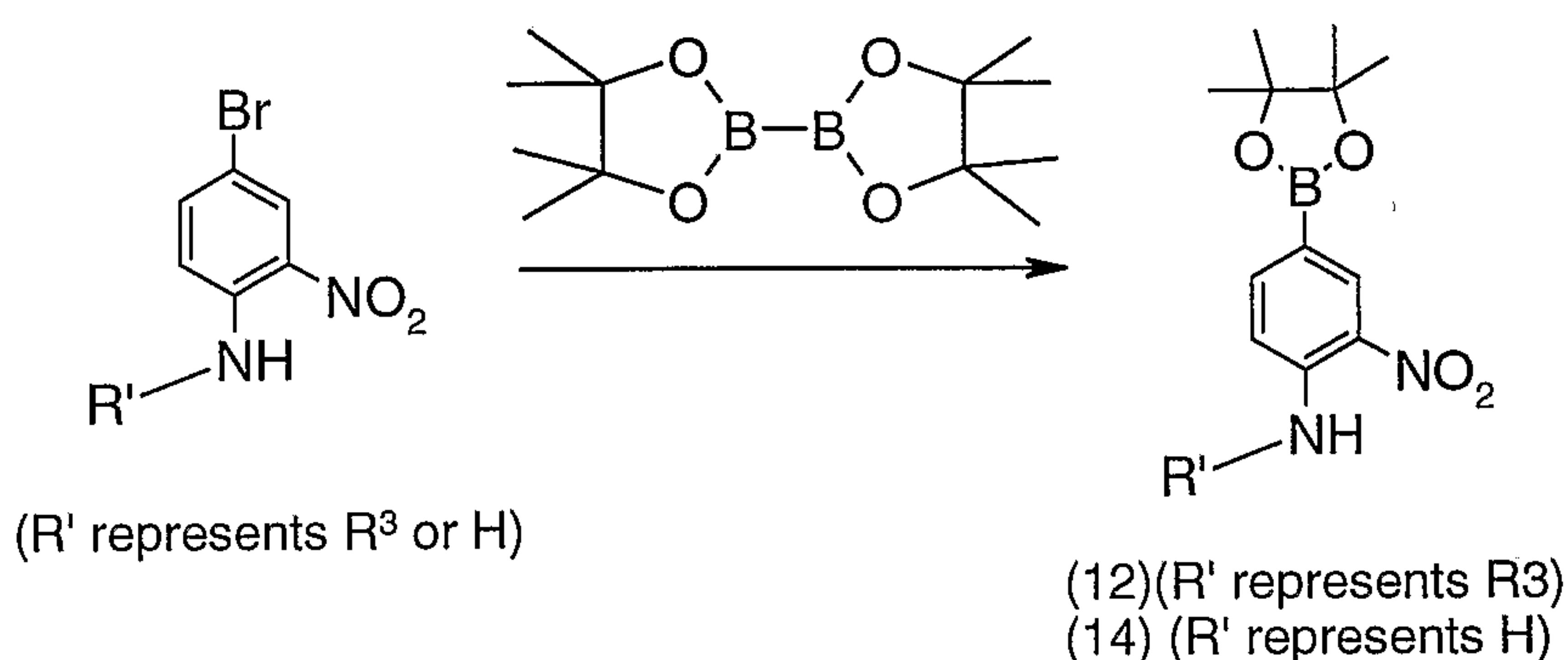
Scheme VI
