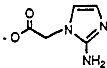
1-carboxymethyl-2-aminoimidazole (I)
