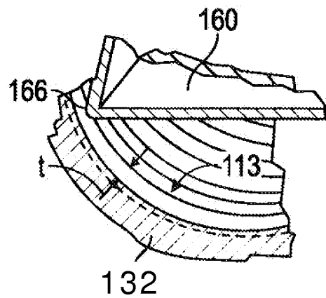
FIG. 6E (Section F-F)
