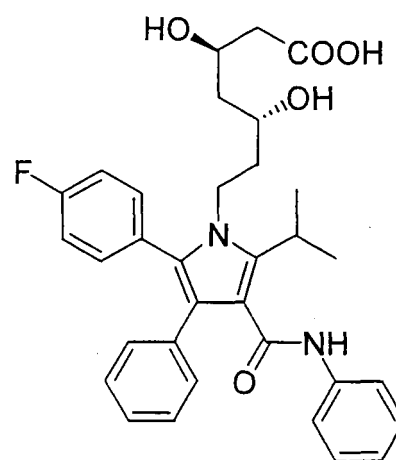
Atorvastatin
