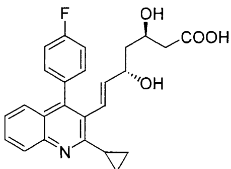
Pitavastatin
