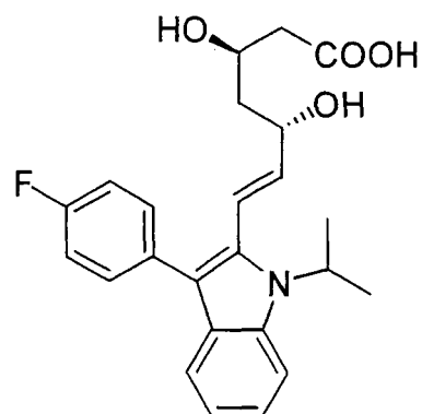
Fluvastatin
