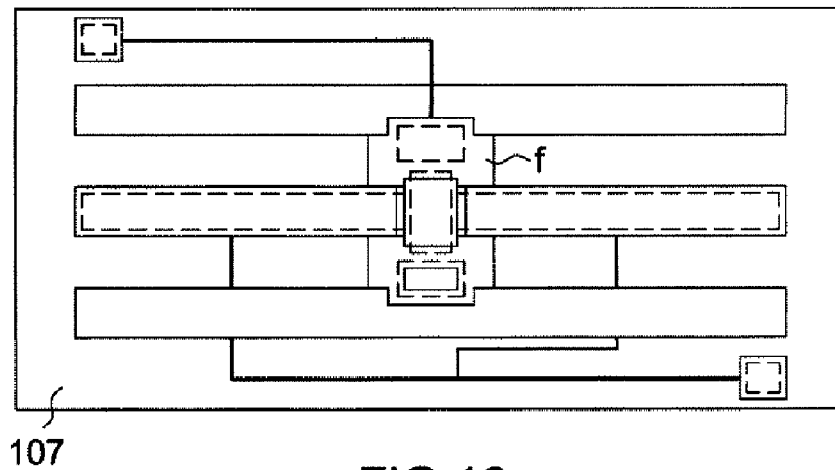
FIG. 16a
