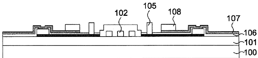
FIG. 16b
