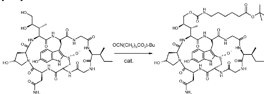
\alpha -amanitin
