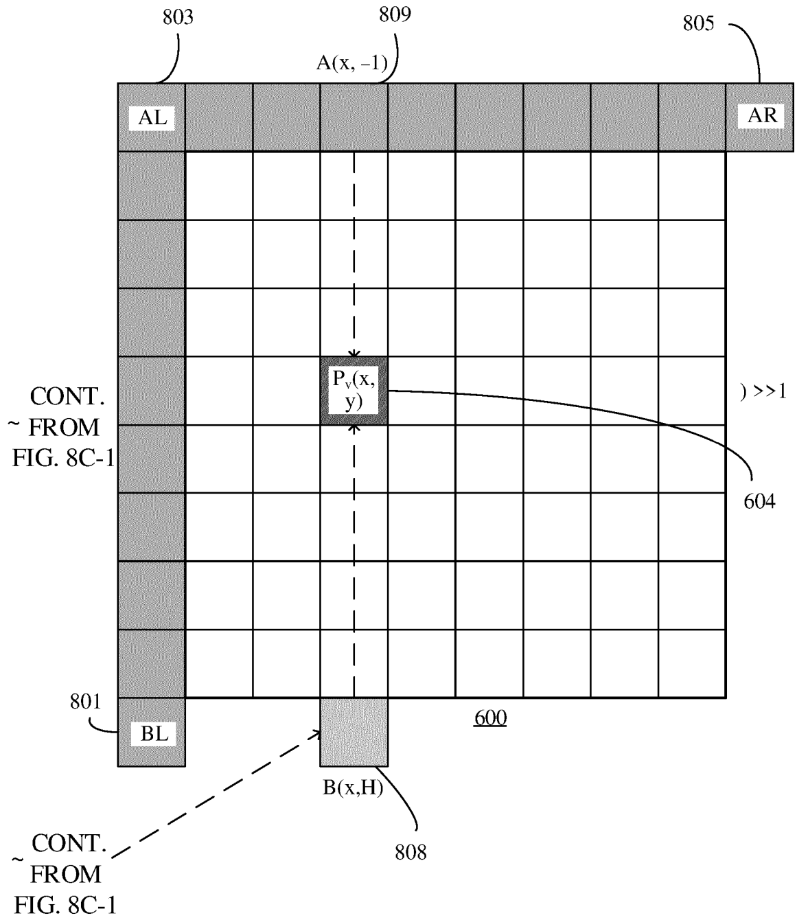
FIG. 8C-2
