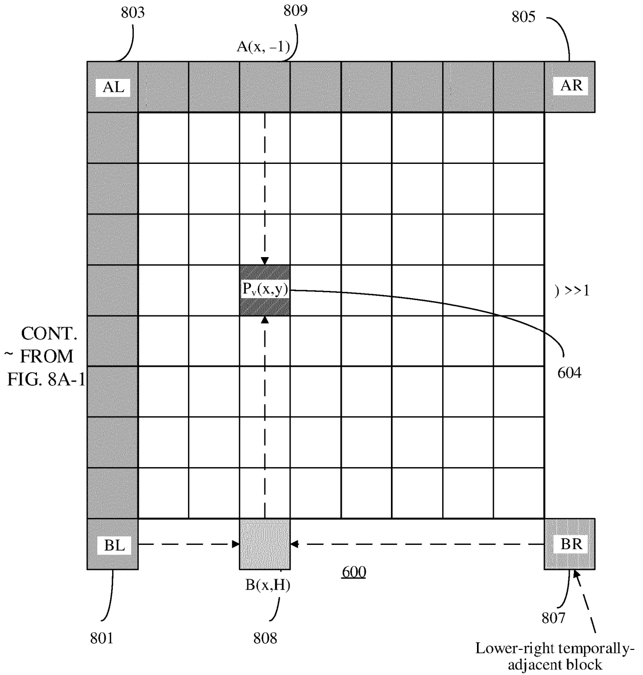
FIG. 8A-2
