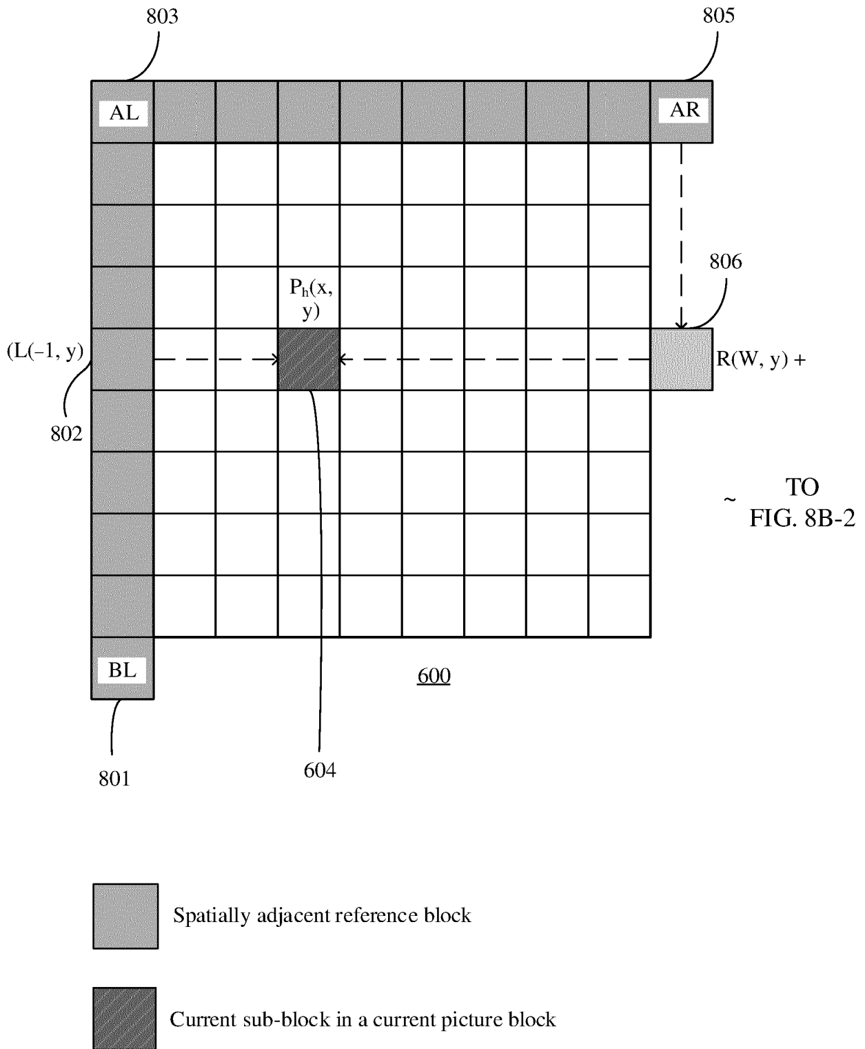
FIG. 8B-1
