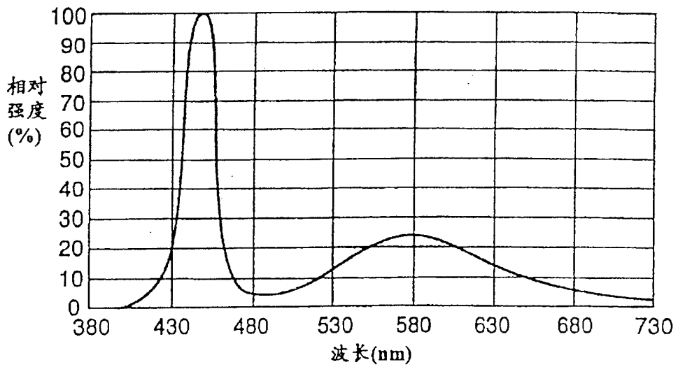
图 19C
