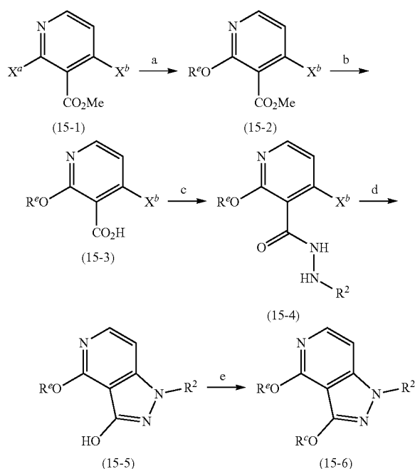
(Scheme 15)
