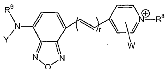
(IXa)
