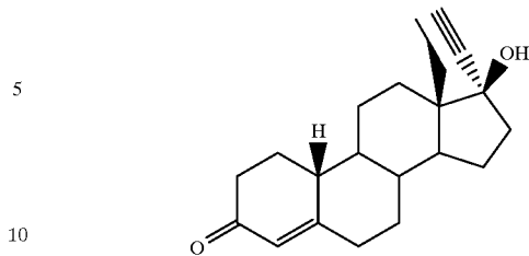
NORGESTREL
