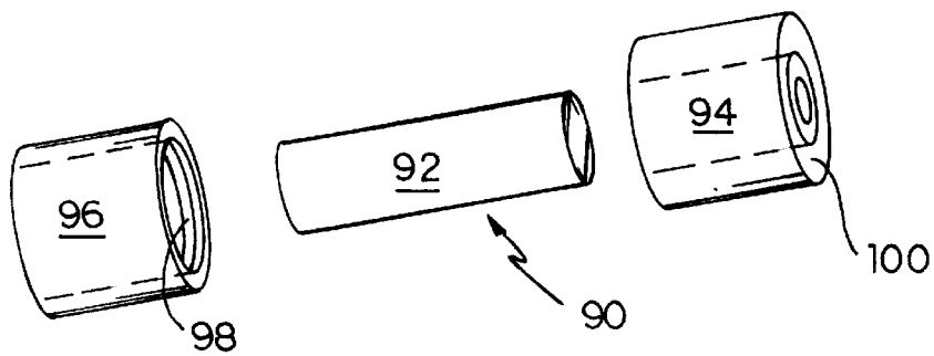
FIG. 7E
